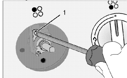
1 Stelschroef gasdebiet
