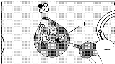
1 Gasdurchfluss-Einstellschraube
