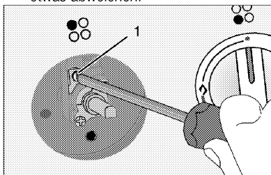
1 Gasdurchfluss-Einstellschraube
